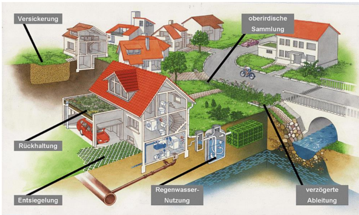
Abbildung 4: Naturnaher Umgang mit Niederschlagswasser – Insbesondere bei der derzeit häufig durchgeführten Nachverdichtung von Siedlungsräumen muss die Niederschlagswasserbeseitigung frühzeitig berücksichtigt werden, ansonsten sind vollgelaufene Keller bei Niederschlägen an der Tagesordnung (weiter Informationen zum Thema Umgang mit Niederschlagswasser unter www.lfu.bayern.de/wasser/niederschlagswasser_umgang/index.htm )
